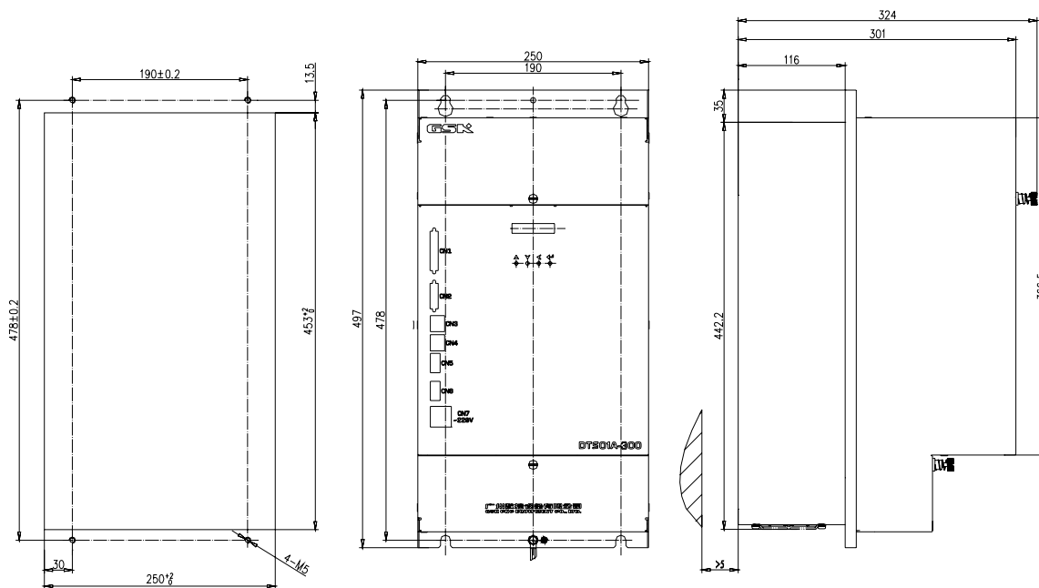
图 2-1 (e) DTS01A-300 开口尺寸图
