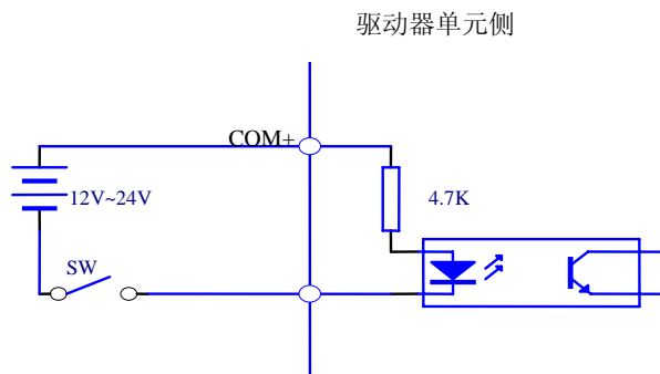
图 3-7 Type1 开关量输入接口
