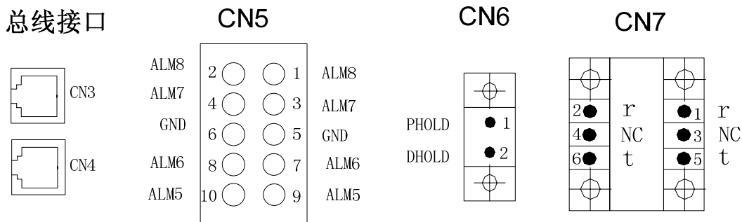
图 3-6 其它端子图
