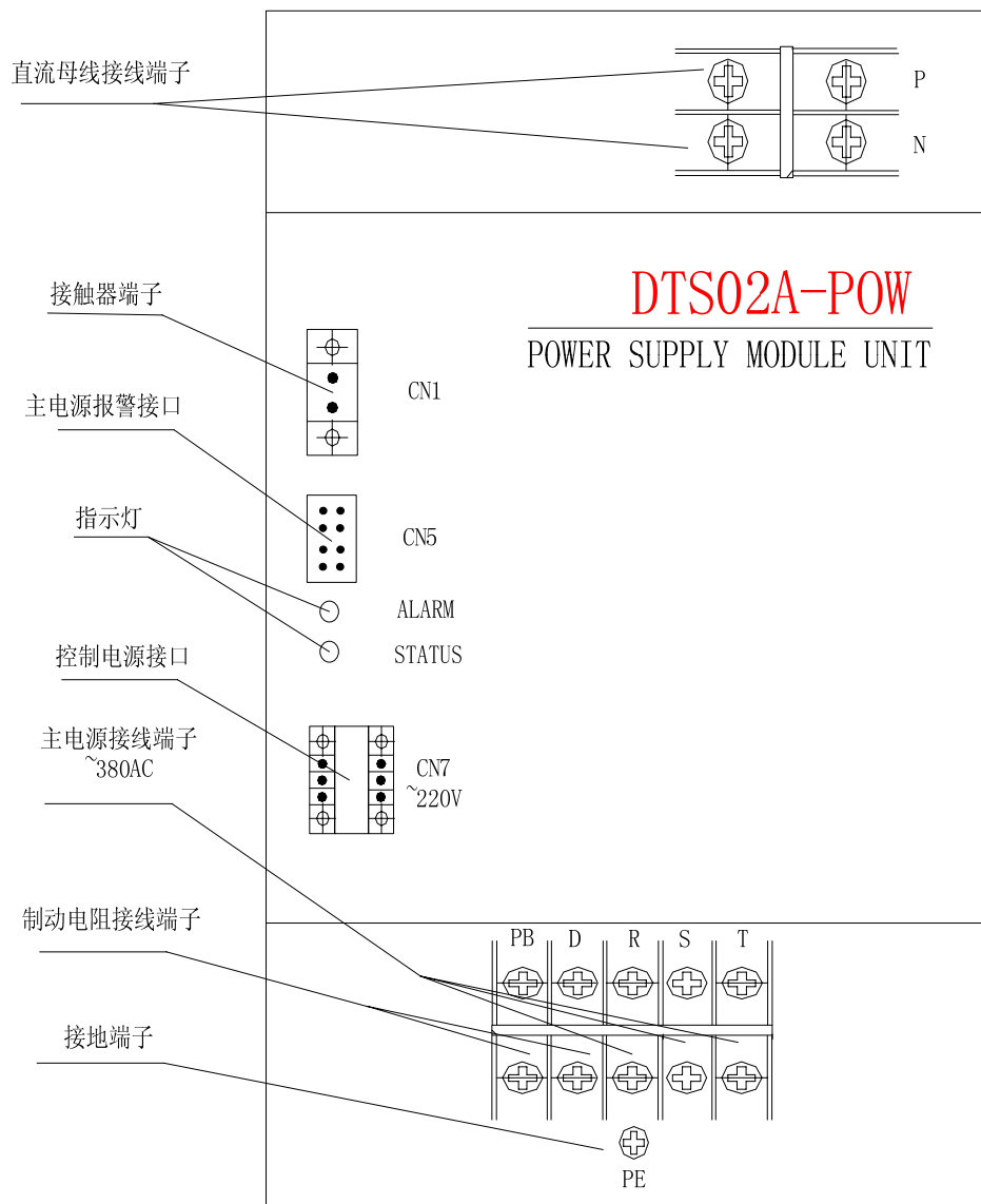
图 1-1 AE-80 全电动注塑机电源模块外观图
