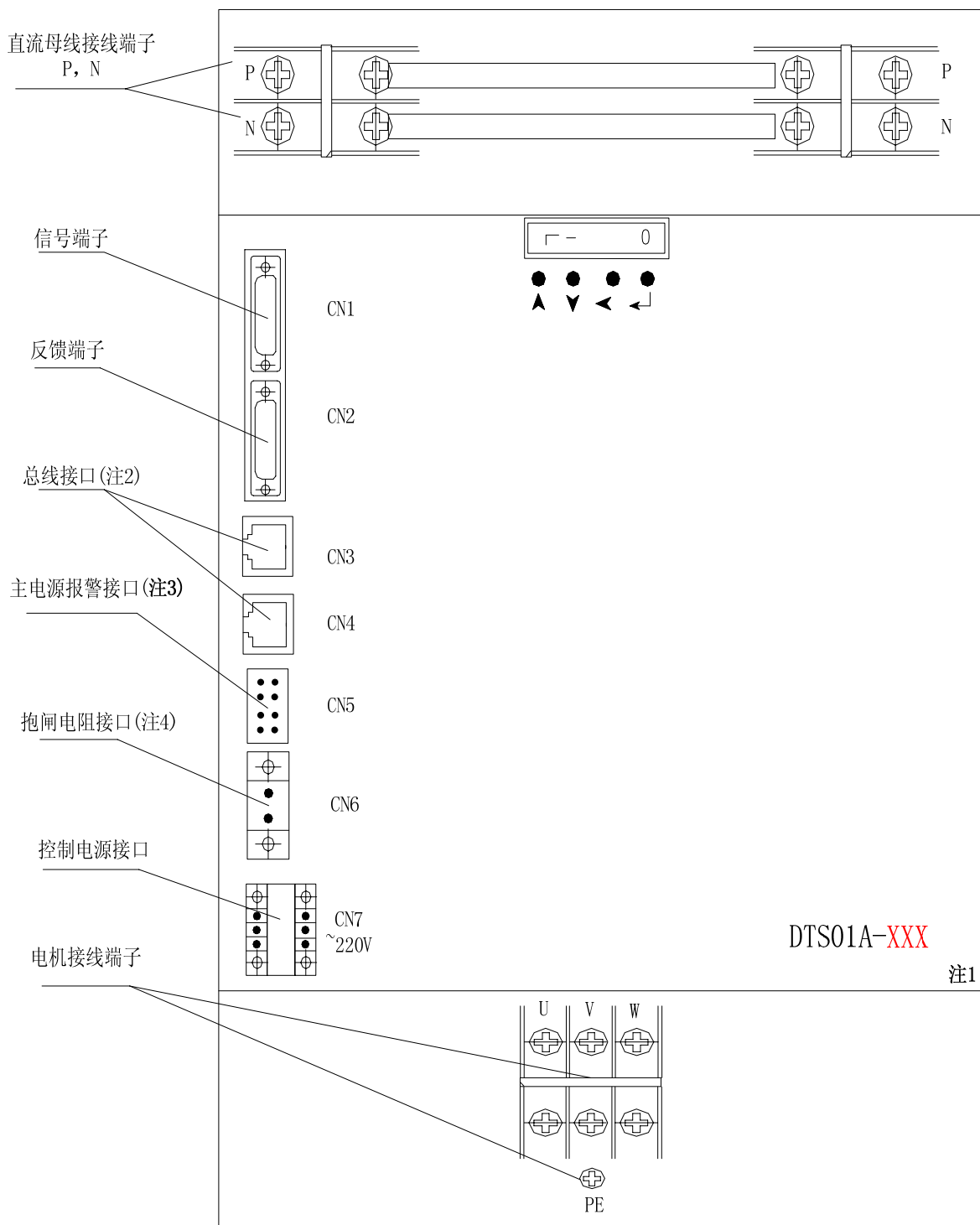
图 1-2 AE-80 全电动注塑机驱动模块外观图
