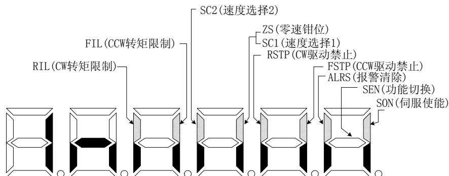
图 6-3 输入端子显示(笔划点亮表示 ON, 熄灭表示 OFF)
