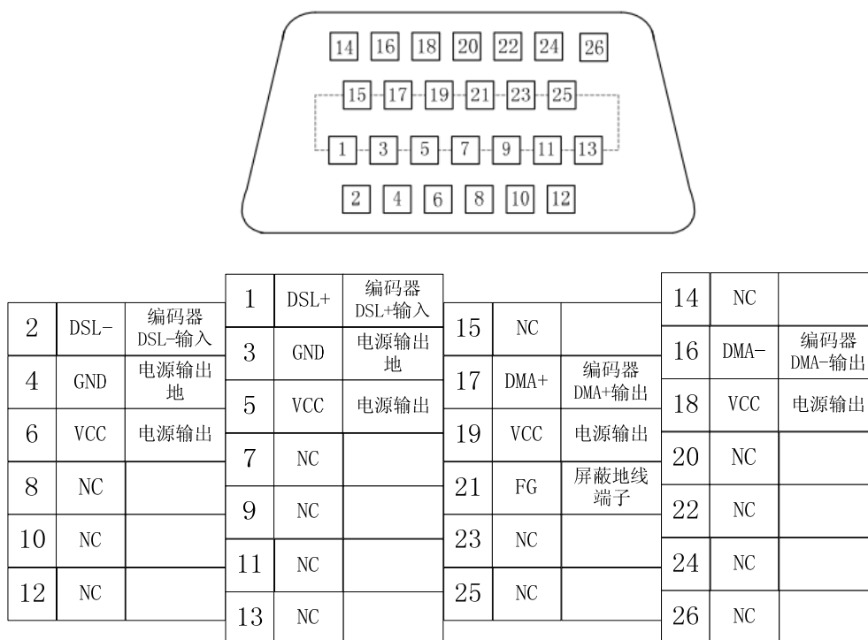
图 3-5 CN2 引脚图
