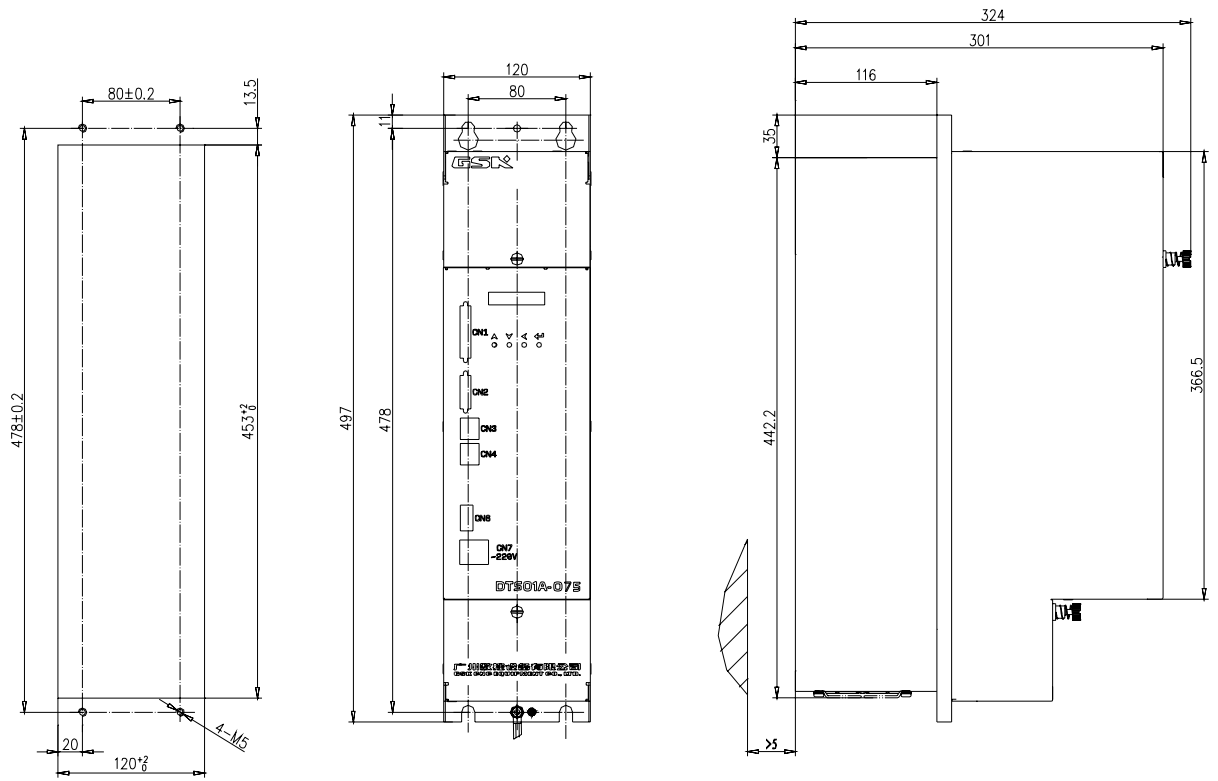
图 2-1 (c) DTS01A-75 开口尺寸图
