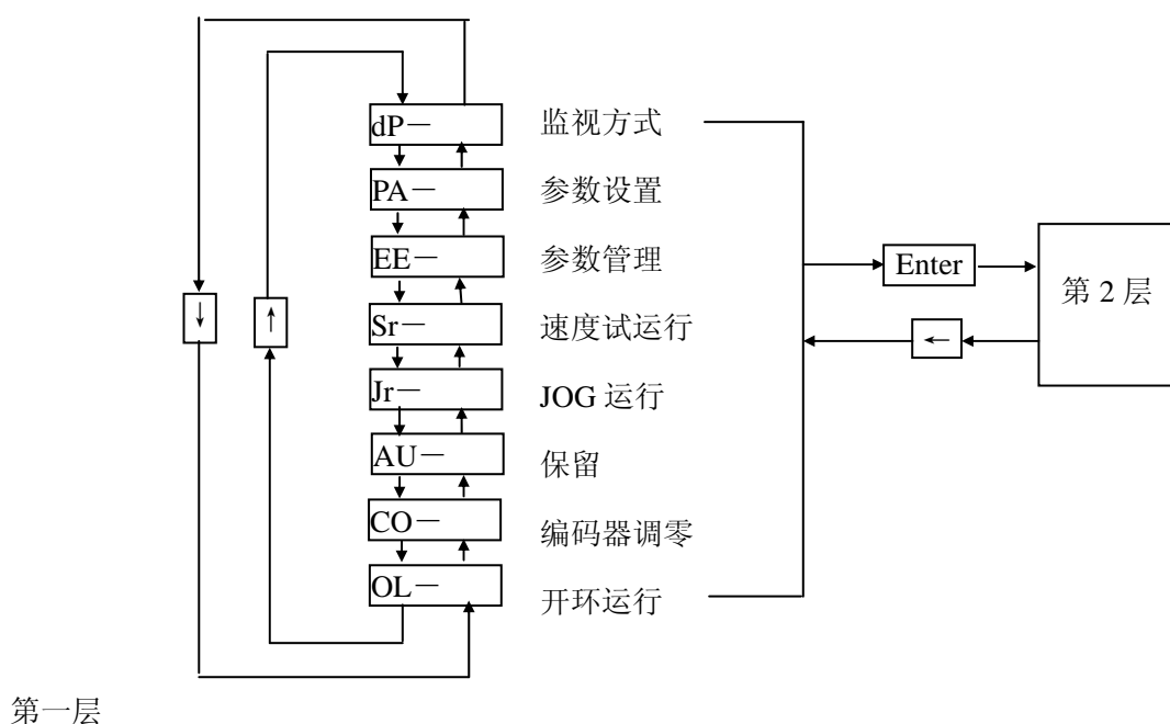
图 6-1 方式选择操作框图
