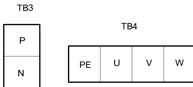
图 3-3 驱动模块中电源端子图
