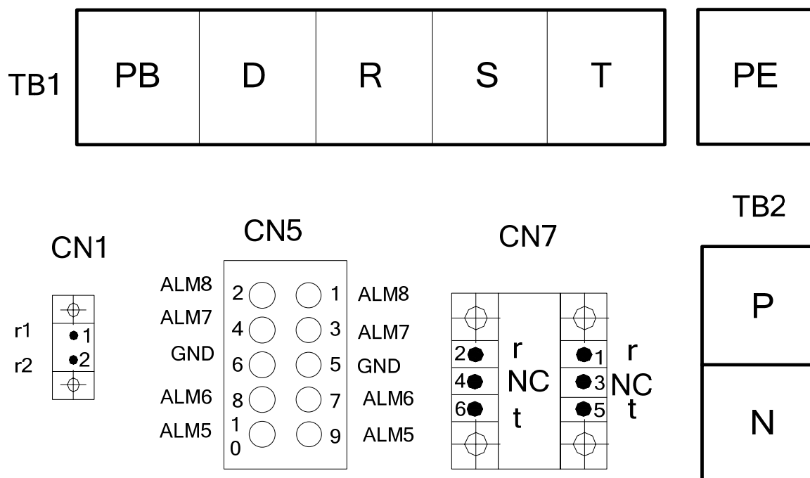
图 3-1 DTS02A-POW 电端子图
