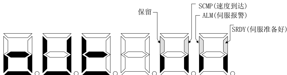
图 6-4 输出端子显示(笔划点亮表示 ON, 熄灭表示 OFF)
