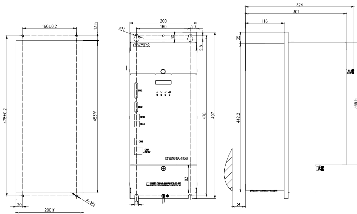
图 2-1 (d) DTS01A-100 开口尺寸图
